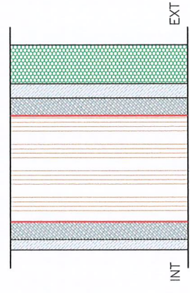
M1 - MURO VERSO ESTERNO NUOVO
